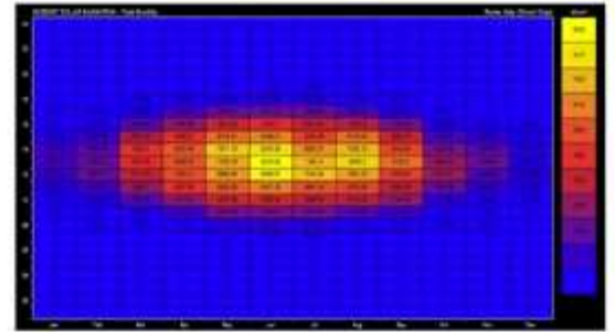
Radiazione solare incidente cumulata mensile (Wh/mq)
