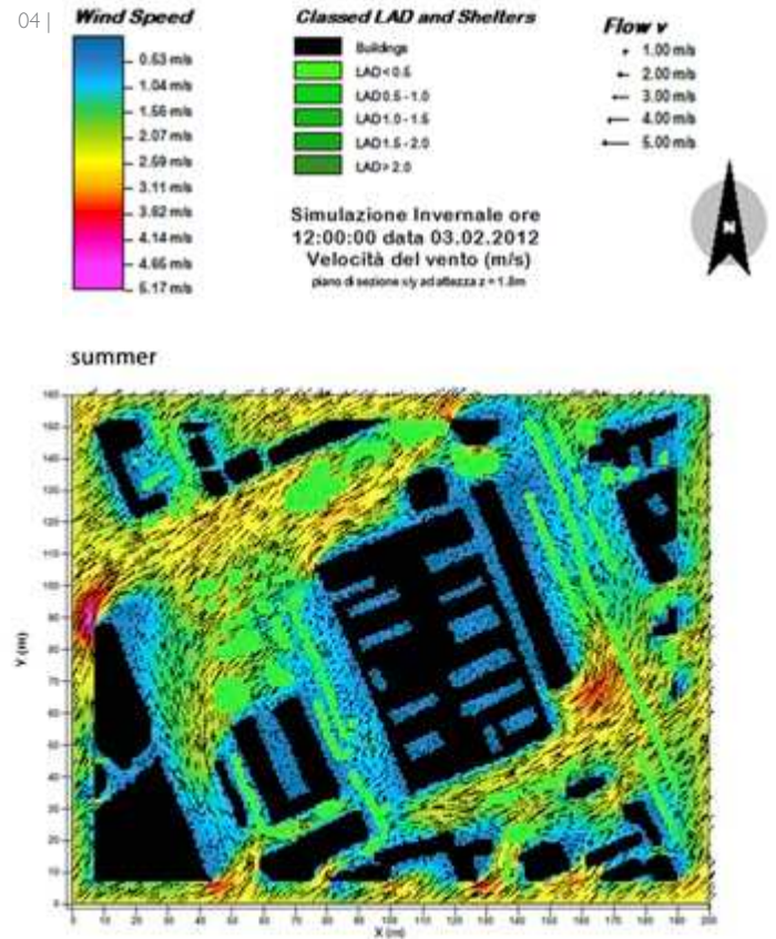
04 | BNCR, una volta analizzate le informazioni generali relative alla condizione climatica del luogo, si è proceduto alla simulazione della ventilazione sull'area urbana e sul volume esterno dell'edificio con il software Envmimet BNCR, once analyzed the general information about the climatic condition of the place, we proceeded to the simulation of the ventilation on the urban area and on the outer volume of the building with the software Envmimet
